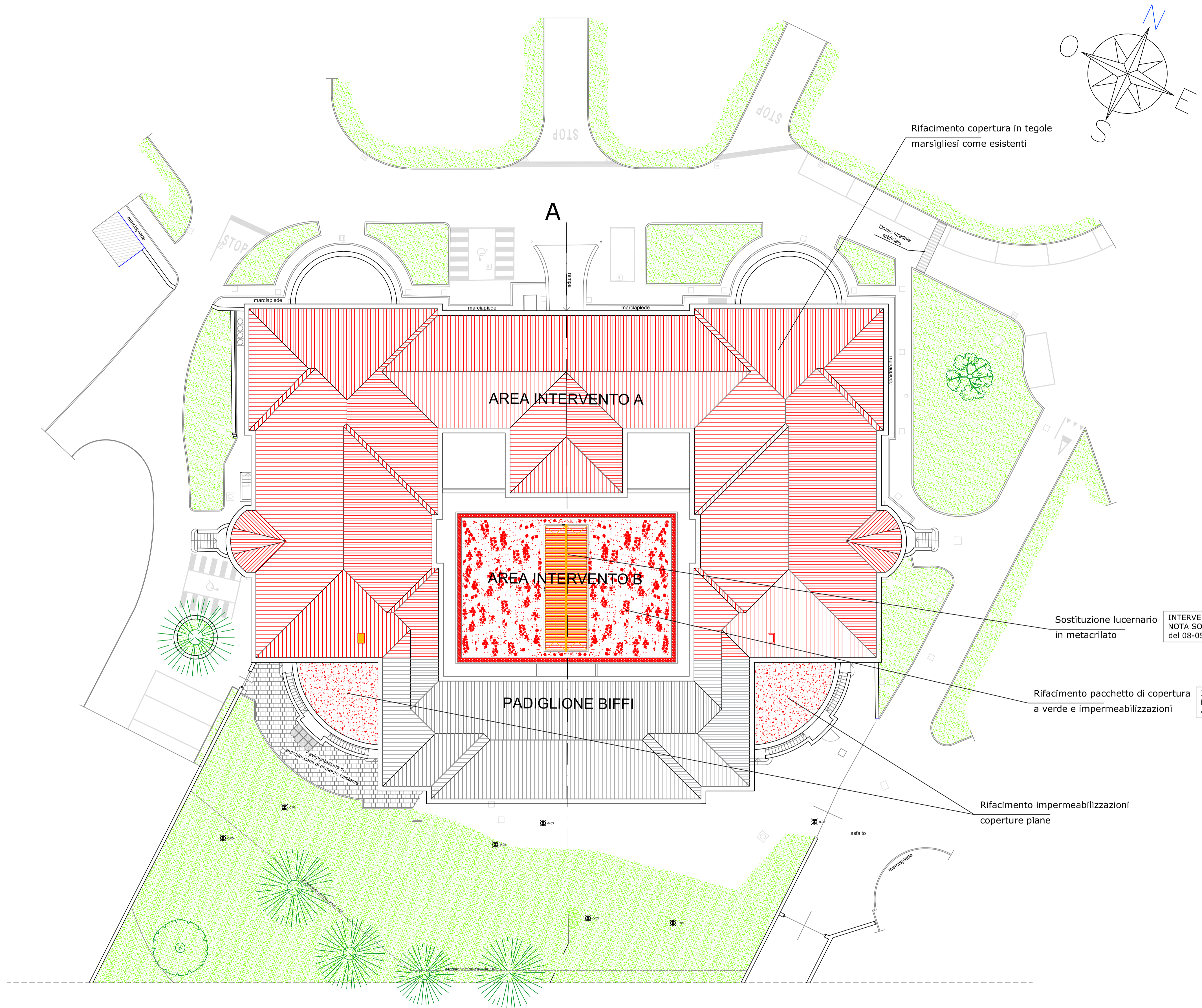
Planimetria generale Raffronto Scala 1:200
